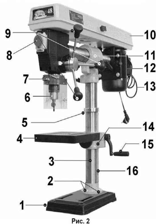
6. УСТРОЙСТВО СТАНКА
